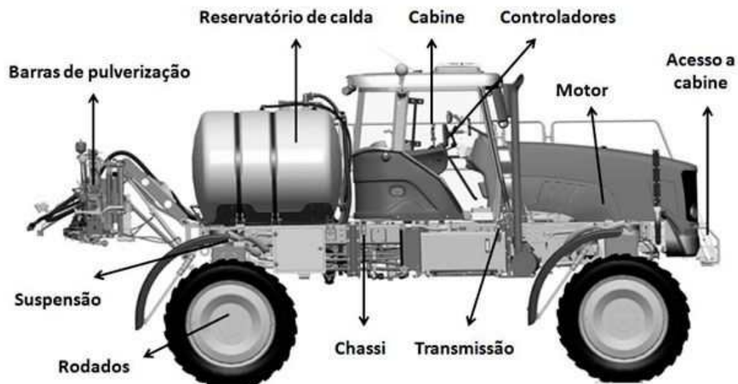
Figura 15. Partes de um pulverizador autopropelido.
