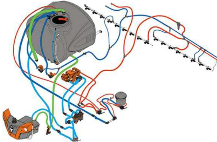
Figura 13. Esquema de sistema de pulverização de um pulverizador autopropelido.
