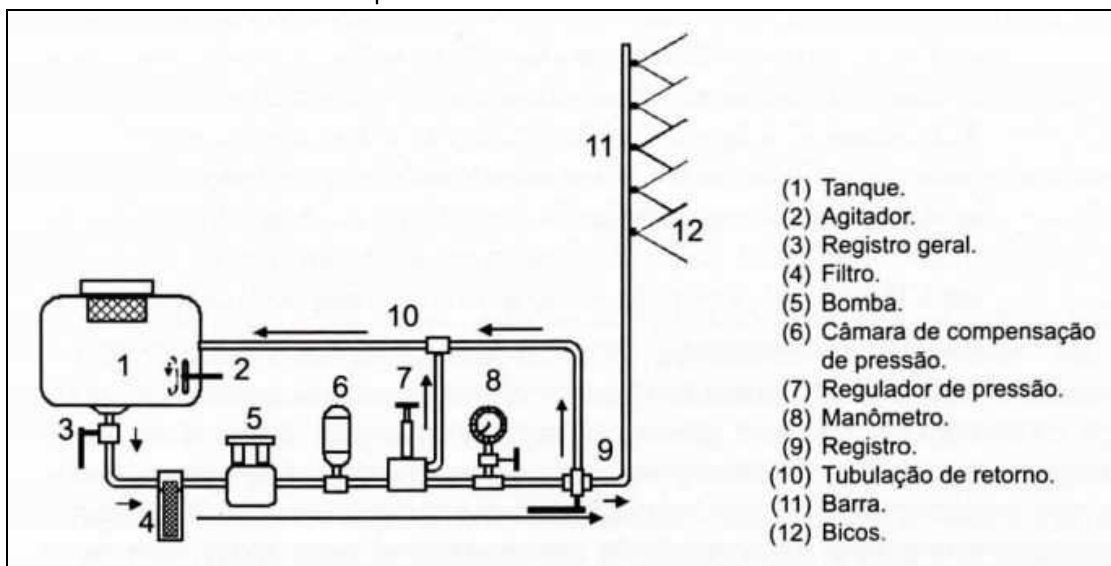
Figura 12. Circuito hidráulico de um pulverizador de barra.
