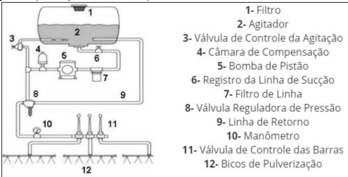
Figura 8. Representação do sistema de um pulverizador.
